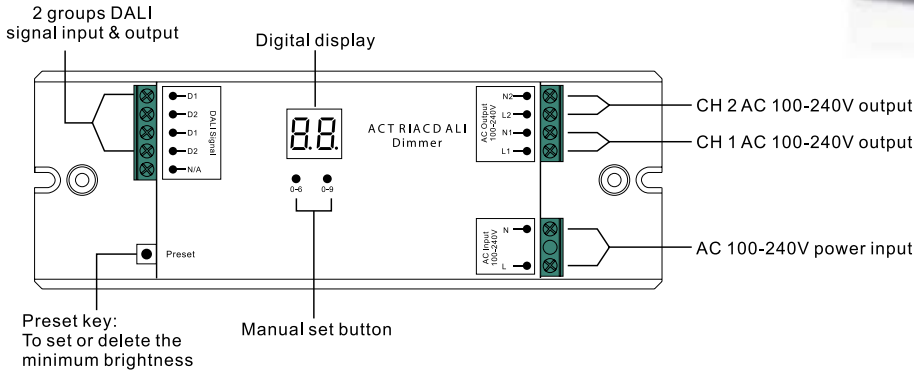
DALI DIMMER LC-2303AC
