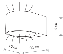
NEL LED painted aluminum, glass
