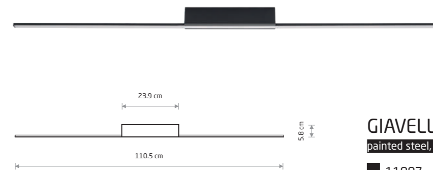
GIAVELLOTTO LED M 11887
